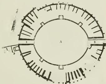
91. sz. Az aquinumi amphitheatrum alaprajza: A) a kuzdótér (arena); B) a kuzdótérre vezető kapuk (portae), és pedig a keleti a p. pompae, melyen a gladiátorok a játék kezdetekor bevonultak, a nyugoti a p. triumphalis, a merre a győztesek elhagyták a kuzdótérrel. 1., 3—6. zárkák a vadállatok számára (carceres), 2. zárka az elesettek testének kivite'ere (porta libitinae); C) nézőtér (cavea). Korszusky I. m. 13. lap után.
